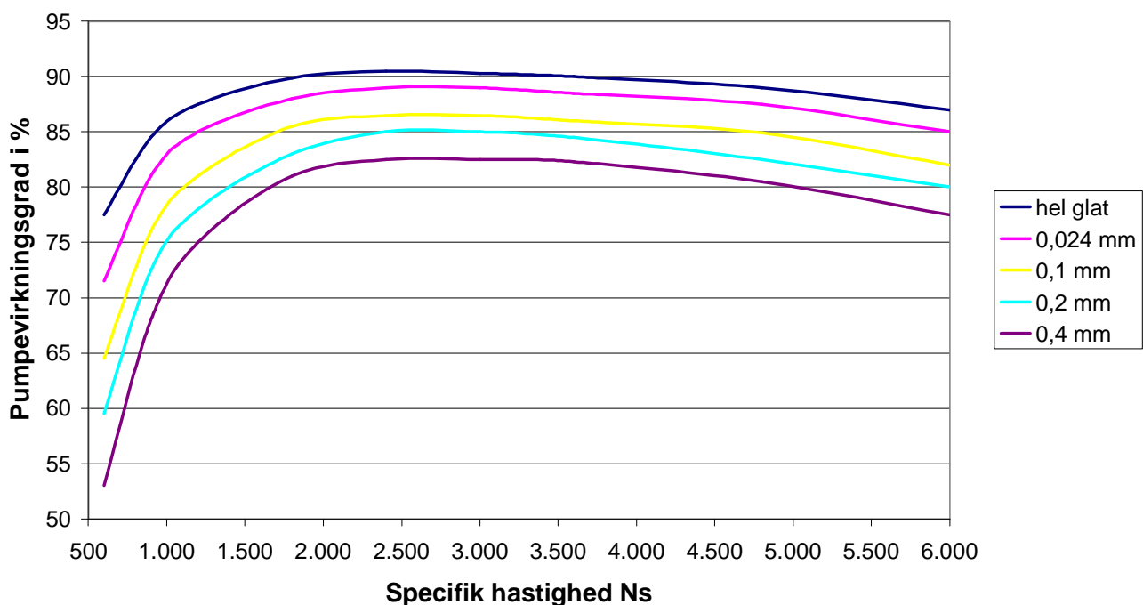
Pumpevirkningsgrad i afhængighed af ruhed
